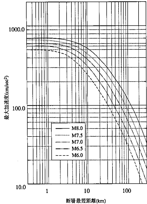
Fig. 2 1種地盤における最大加速度の距離減衰特性 Maximum Acceleration from Earthquake Fault for No.1 Ground Type
