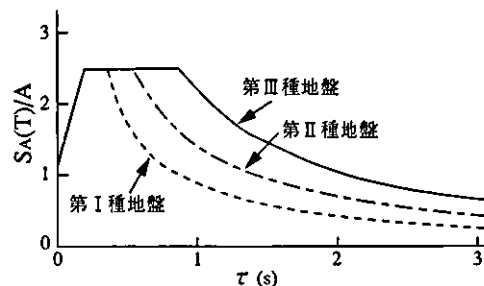
Fig. 3 地盤種別ごとの水平動基準化加速度応答スペクトル Maximum Response Acceleration Spectrum to Horizontal Ground Motion
