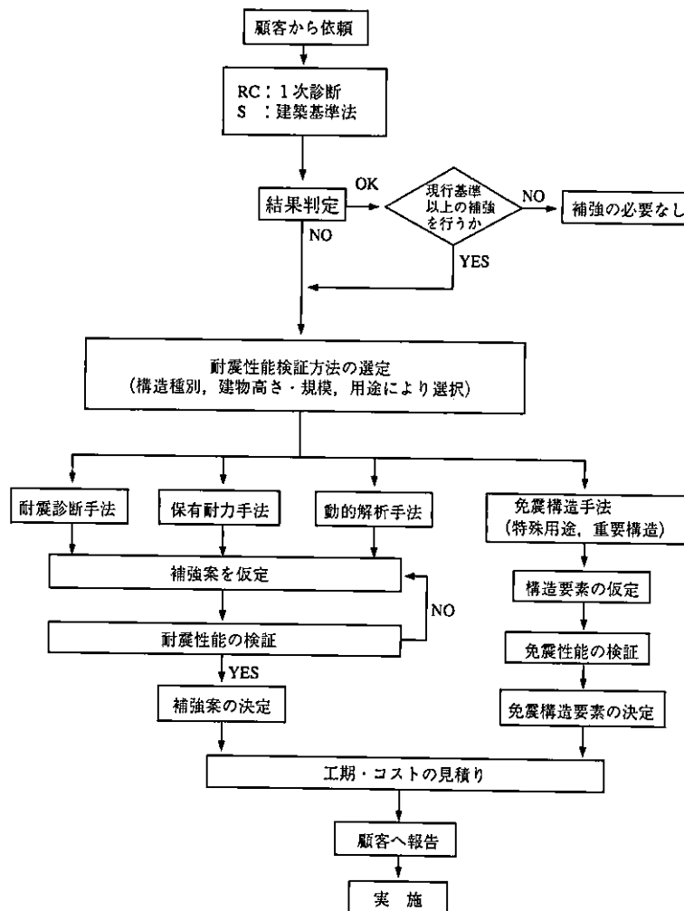
Fig. 1 補強計画のフロー Flow Diagram of Retrofitting Procedure
